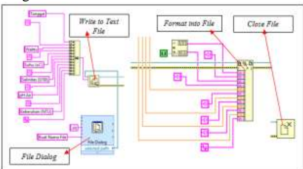
Gambar 15. Program Penyimpanan Data Pada LabVIEW
