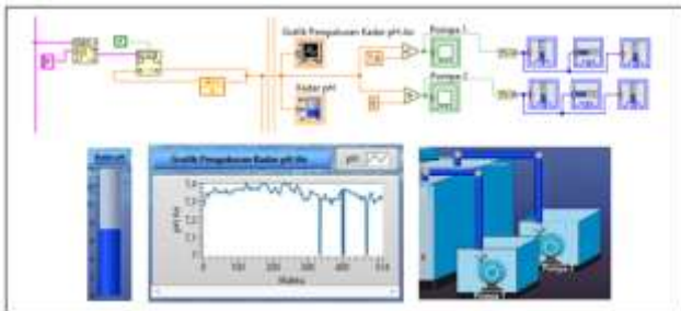
Gambar 13. Program Tampilan Pengontrolan pH pada Perangkat Lunak LabVIEW
