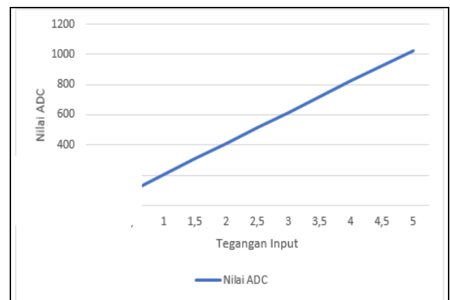
Gambar 7. Hubungan Input Tegangan Terhadap ADC
