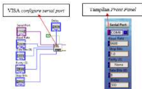
Gambar 8. Konfigurasi Serial Data Program LabVIEW
