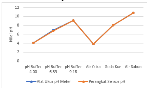
Gambar 5. Kalibrasi Nilai Sensor pH Terhadap Alat Ukur Standar pH Meter
