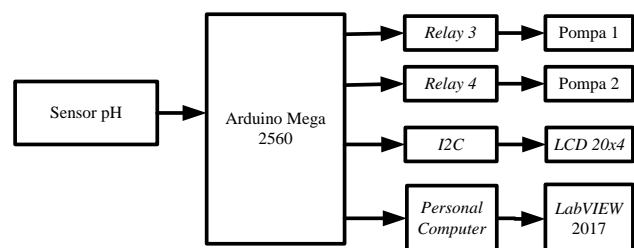
Gambar 1. Blok Diagram Perancangan Perangkat
