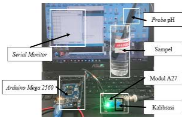
Gambar 4. Pembacaan Sensor pH Melalui Serial Monitor
