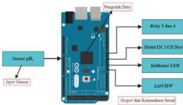
Gambar 2. Perancangan Perangkat Keseluruhan
