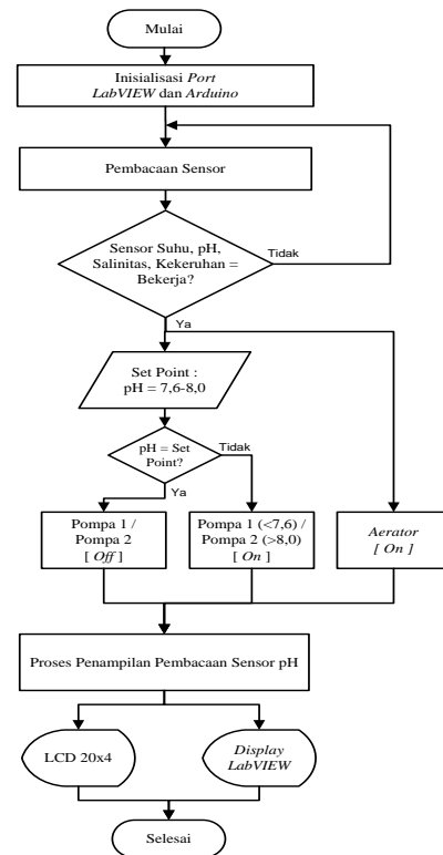
Gambar 3. Diagram Alir Cara Kerja Sistem Perangkat
