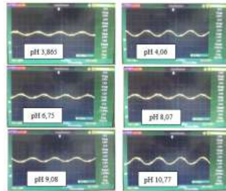
Gambar 6. Pengujian Sensor pH Menggunakan Osiloskop
