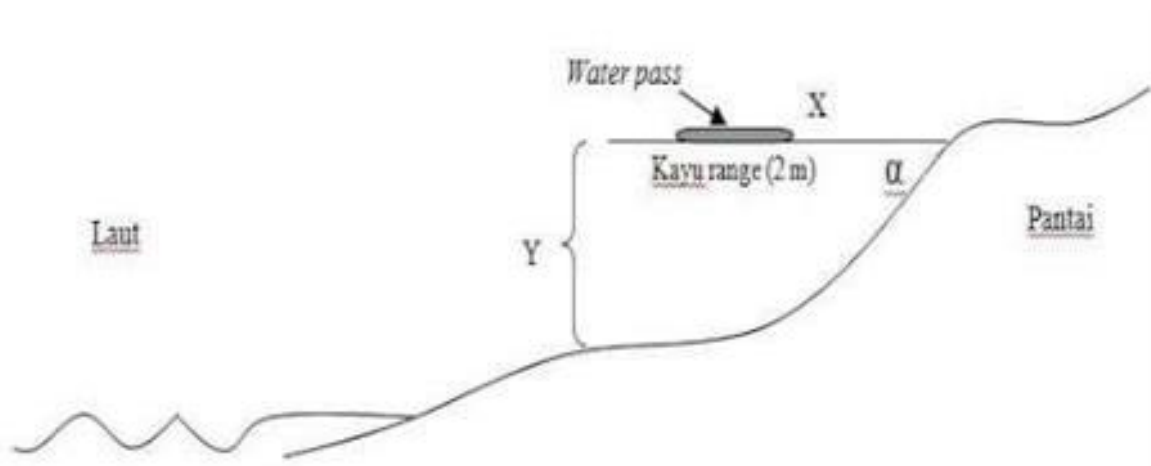
Gambar 2. Pengukuran kemiringan pantai
